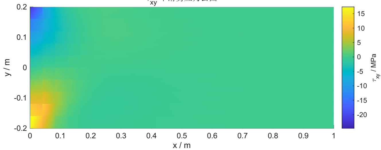
\tau_{xy} 平滑剪应力云图
